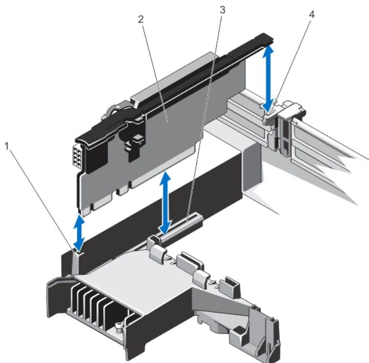
Ilustración 30. Extracción e instalación de la tarjeta vertical de expansión 3
