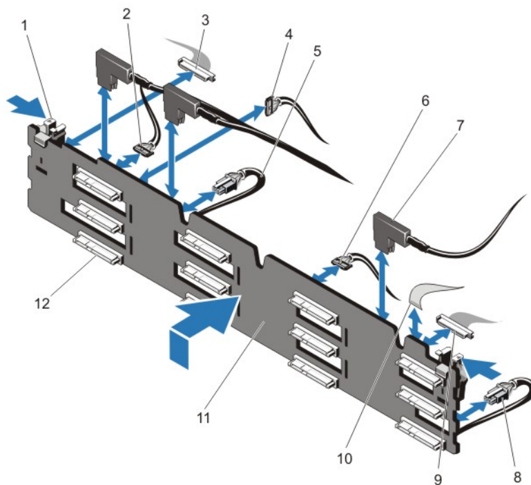
Ilustración 40. Extracción e instalación del plano posterior SAS (x12) de 3,5 pulgadas
