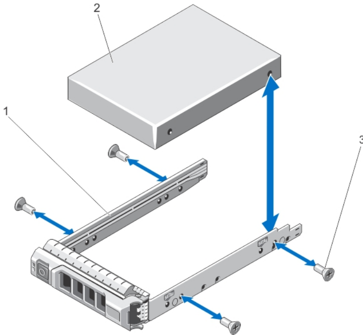
Ilustración 17. Extracción e instalación de una unidad de disco duro en un portaunidades de disco duro
