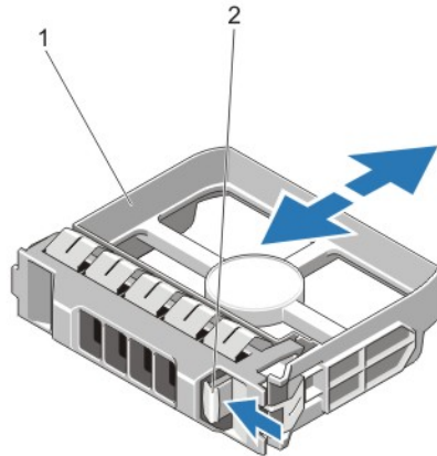
Ilustración 15. Extracción de una unidad de disco duro de relleno de 3,5 pulgadas
