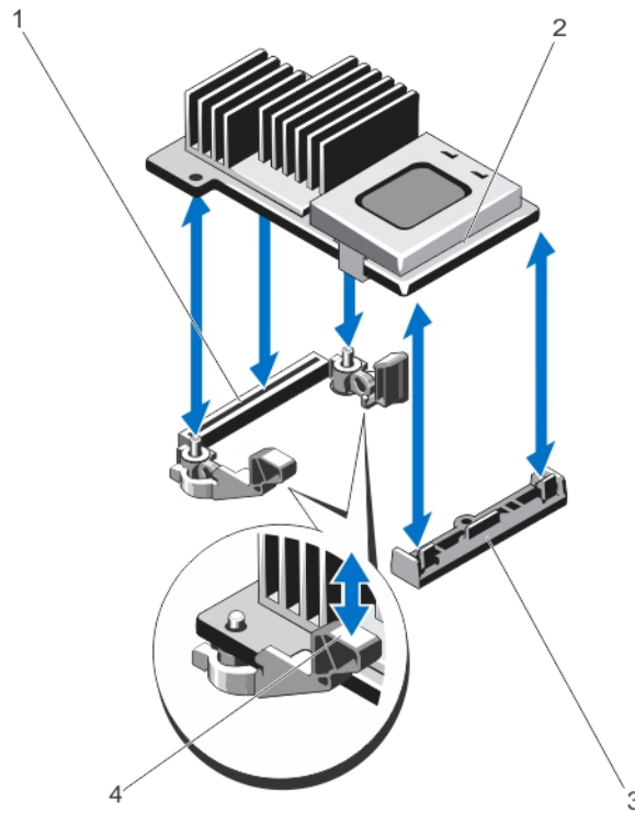
Ilustración 32. Extracción e instalación de la tarjeta controladora de almacenamiento integrada
