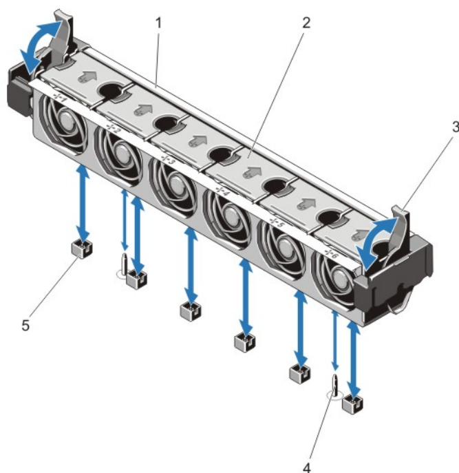
Ilustración 19. Extracción e instalación del conjunto de ventiladores de refrigeración
