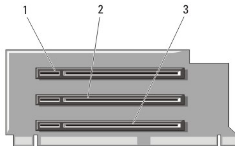
Ilustración 27. Identificación de los conectores del soporte vertical 1 para tarjetas de expansión
