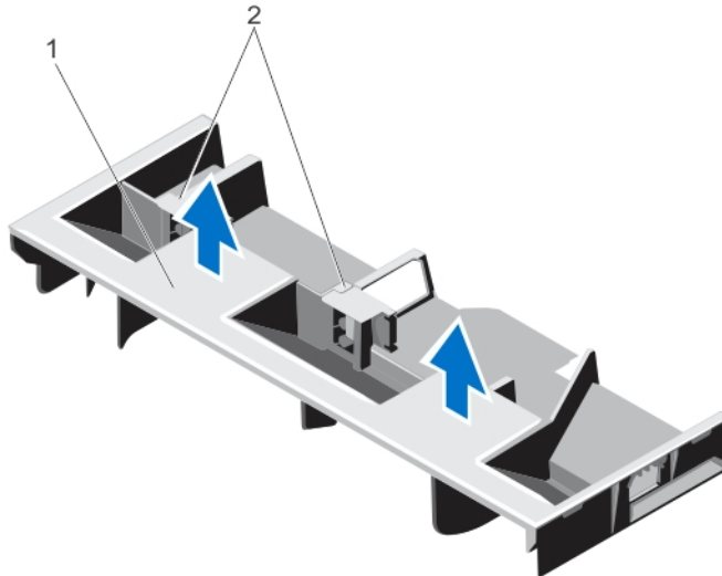
Ilustración 9. Extracción e instalación de la cubierta de refrigeración
