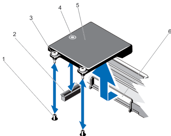
Ilustración 33. Extracción e instalación de una tarjeta secundaria de red
