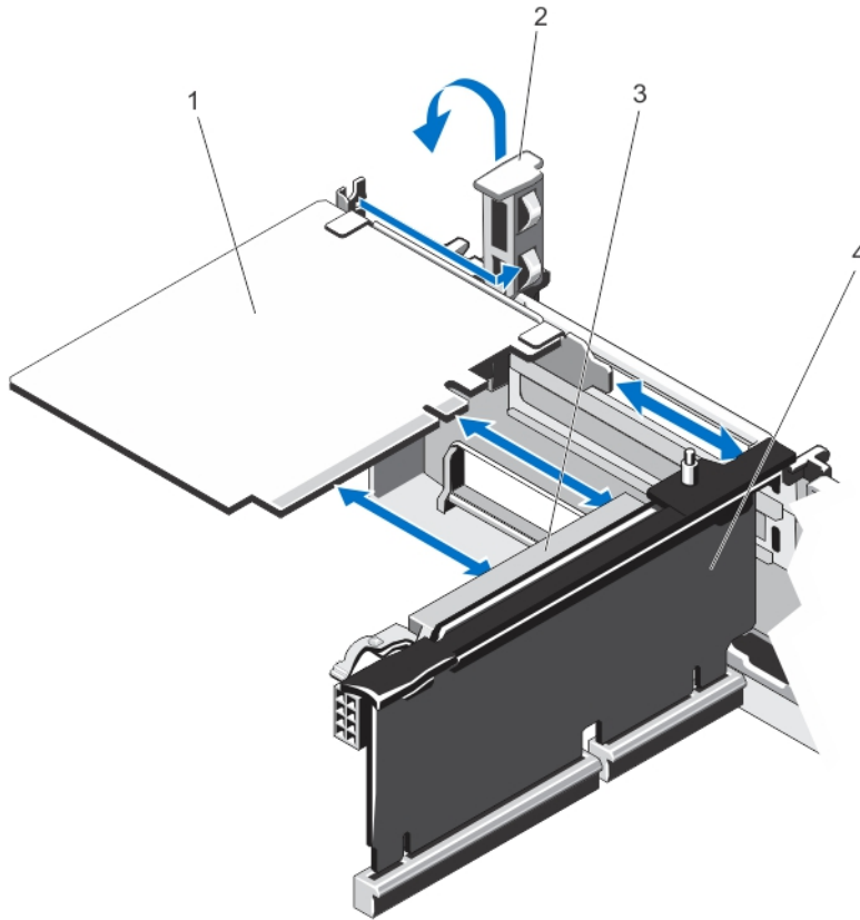
Ilustración 24. Extracción e instalación de la tarjeta de expansión
