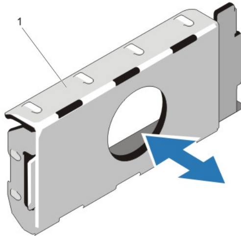
Ilustración 38. Extracción e instalación del panel protector del suministro de energía
