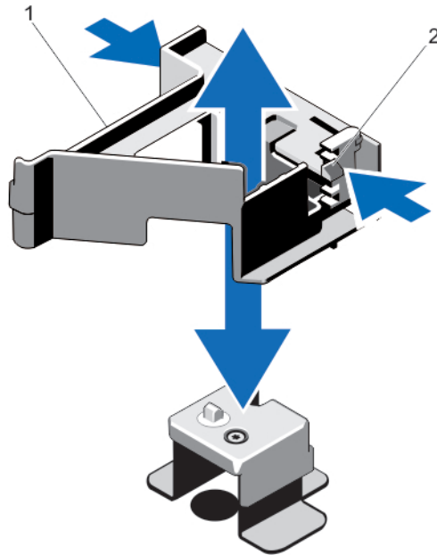
Ilustración 21. Extracción e instalación del soporte para tarjeta PCIe
