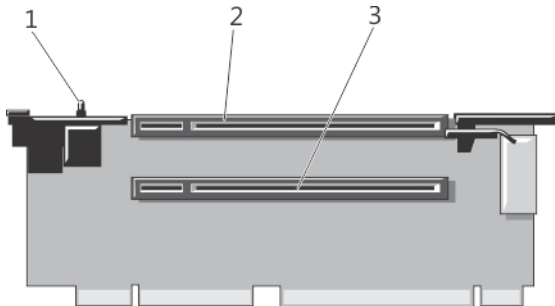
Ilustración 29. Identificación de los conectores del soporte vertical 2 para tarjetas de expansión
