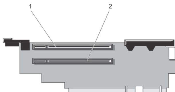
Ilustración 31. Identificación de los conectores del soporte vertical 3 para tarjetas de expansión
