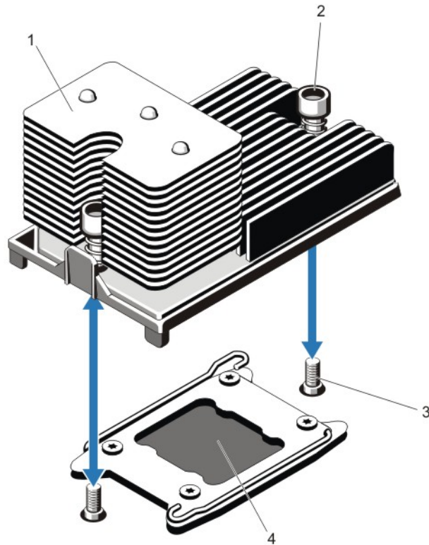
Ilustración 34. Extracción e instalación del disipador de calor del procesador
