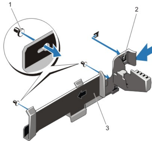
Ilustración 23. Extracción e instalación del soporte de retención de cables
