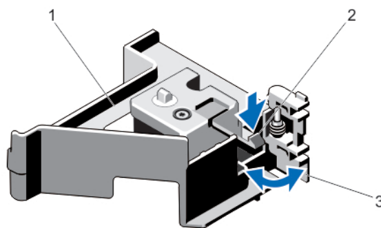
Ilustración 22. Apertura y cierre del pestillo del soporte de tarjeta PCIe
