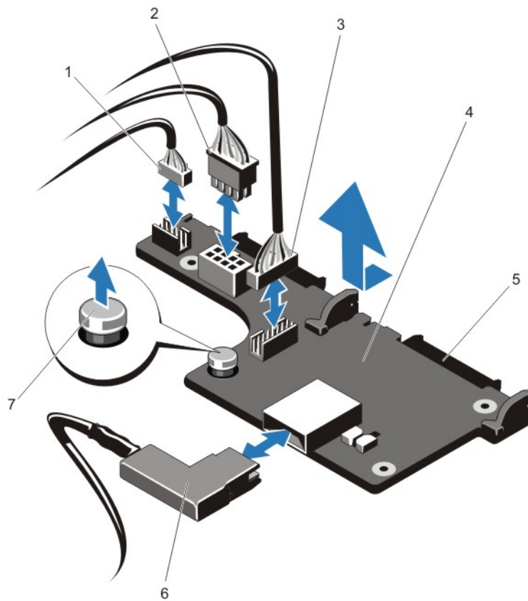
Ilustración 42. Extracción e instalación del plano posterior de la unidad de disco duro (x2) opcional de 2,5 pulgadas
