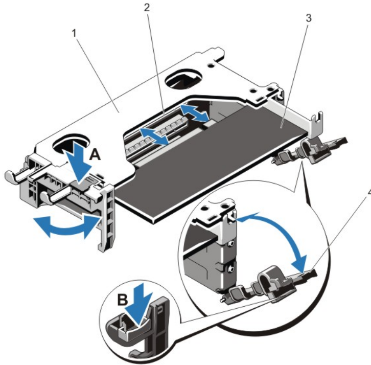
Ilustración 25. Extracción e instalación de la tarjeta vertical de expansión 1
